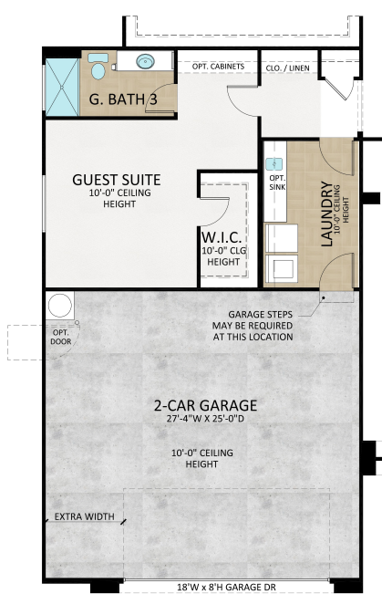
Optional Guest Suite In lieu of Tandem Garage
